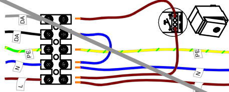
Cablaggio per gestione con pulsante "NA" - Wiring for operation with button "NA" - De cableado para la operación con el botón de "NA" - Câblage pour un fonctionnement avec le bouton "NA" - Verdrahtung für den Betrieb mit Button "NA"
