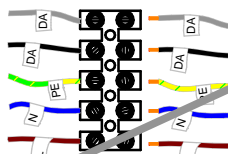
Cablaggio per gestione DALI standard - DALI standard wiring for management - La gestión de cableado estándar DALI - Gestion du câblage standard DALI - Cabling Management DALI-Standard
