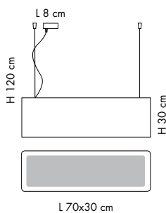
SP 7/501-L 2 x max 70W ECO E27 CE IP20
