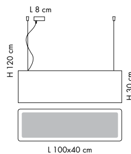
SP 8/501-L 3 x max 70W ECO E27 CE IP20
