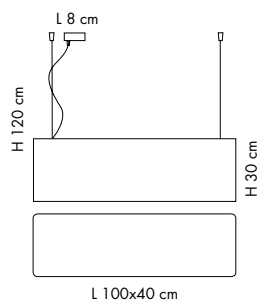
SP 8/501 3 x max 70W ECO E27 CE IP20
