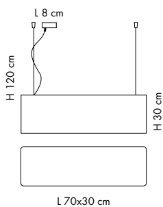
SP 7/501 2 x max 70W ECO E27 CE IP20
