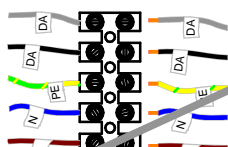
Cablaggio per gestione DALI standard - DALI standard wiring for management - La gestión de cableado estándar DALI - Gestion du cablage standard DALI - Cabling Management DALI-Standard
